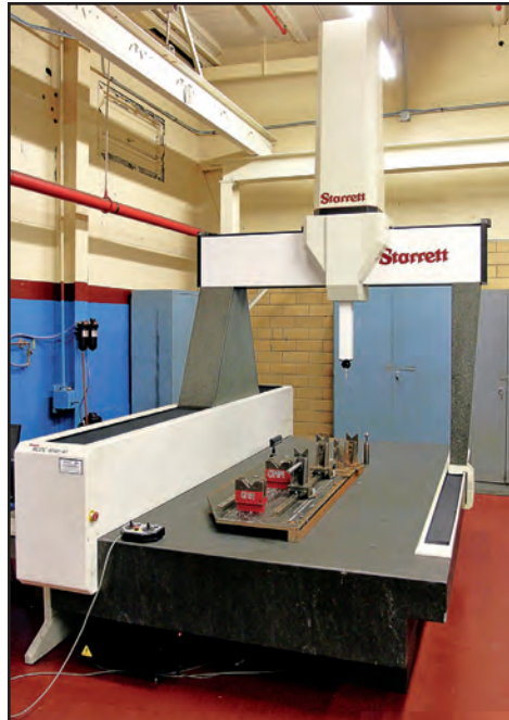
STARRETT RGDC 8048-40 CMM
